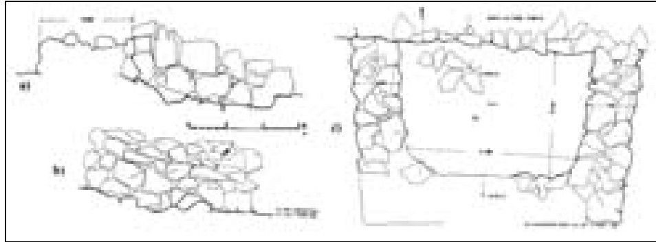
Sl. 5. Struktura pretpovijesnog bedema i kule na gradini Rača (A. Faber)
